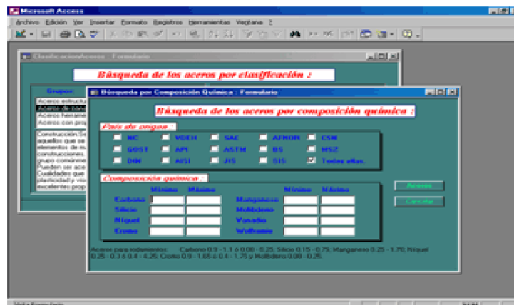
Figura 7. Diálogo de búsqueda de aceros por composición química.
