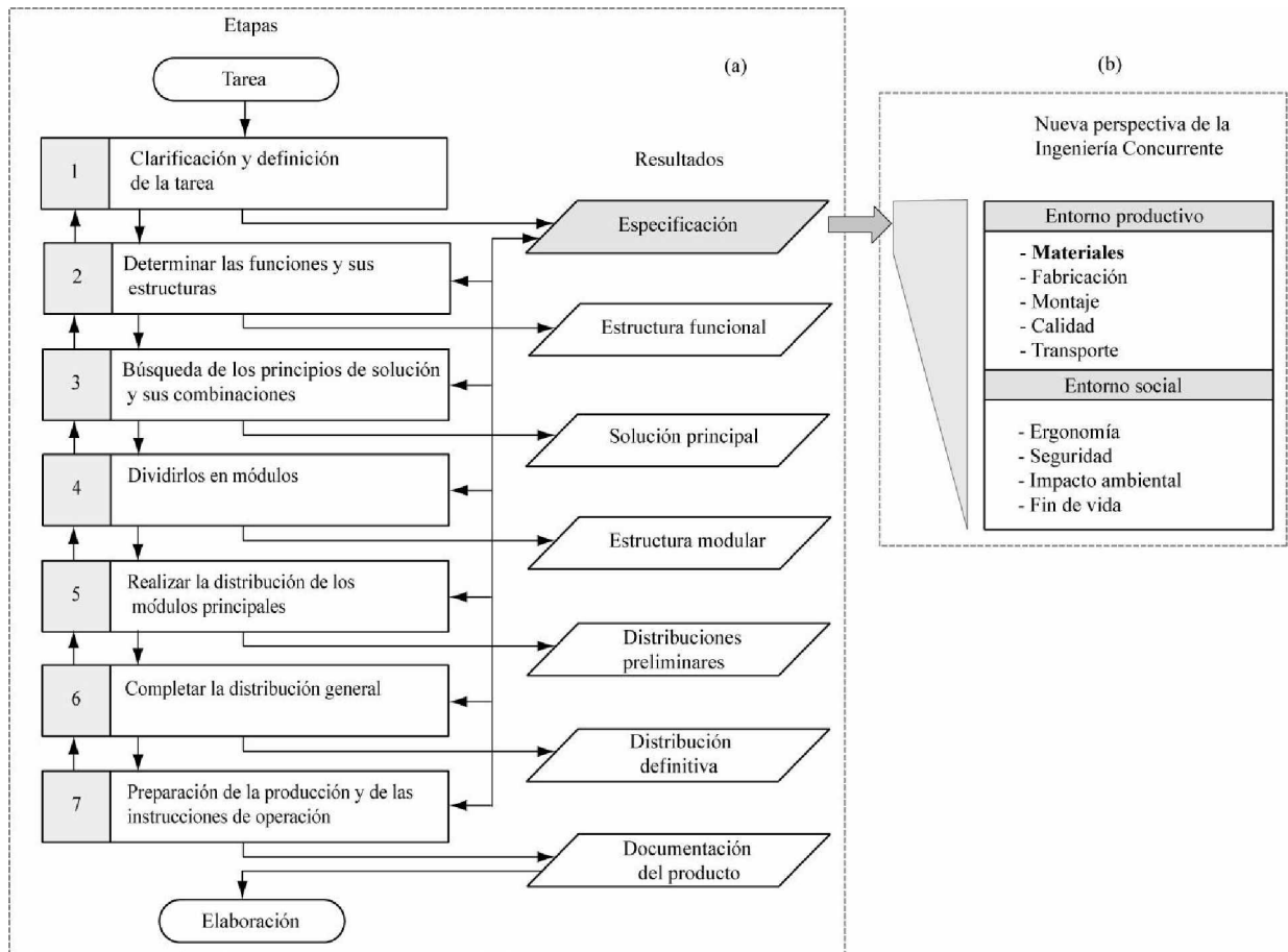
Figura 1. Etapas del proceso de diseño según la norma VDI 2221.
